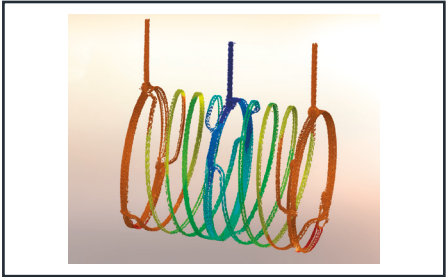
FEM-Simulation der Temperaturverteilung im Rezipienten
