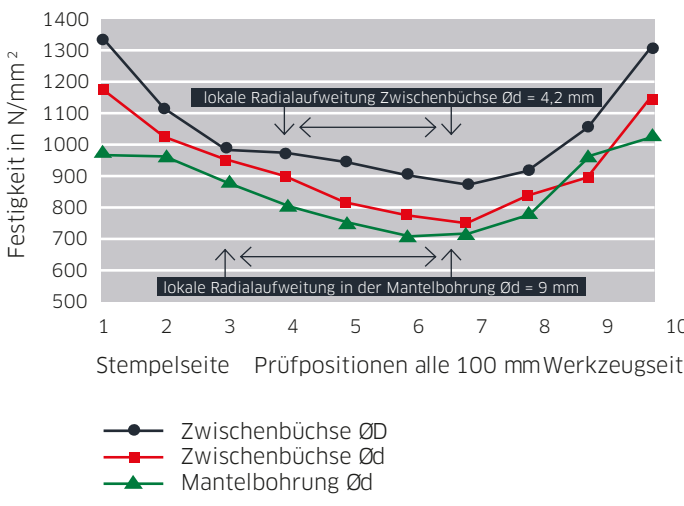
Umstellung des Rezipienten auf Luftkühlung; Verwendung von warmfesten Mantel-Werkstoffen und HTR-Zwischenbüchsen in Kombination mit SA718 Innenbüchsen
