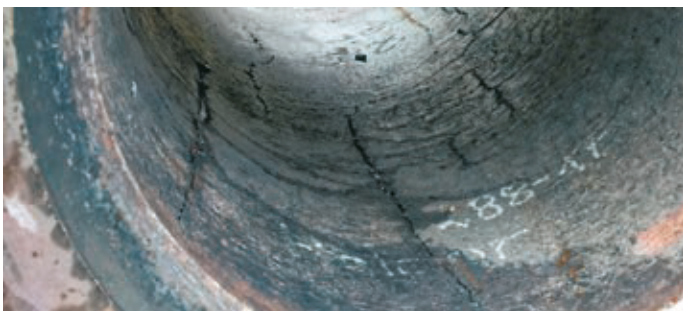
HWF (1000 – 1150 MPa) nach 30.000 Cu-Pressbolzen, grobes Rissnetzwerk mit Ausbrüchen
